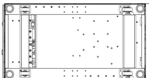
Вид снизу
