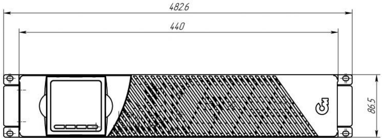
Габаритный чертеж ИБП СИПБ1КА.10-11
